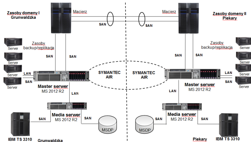
Rys. II.1 Schemat instalacji centralnego systemu archiwizacji aktualnie posiadanego przez Zamawiającego.
