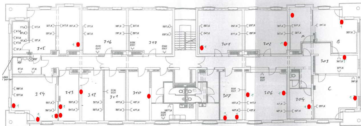
Rys.3 Schemat pomieszczeń na III piętrze z zaznaczonymi (czerwone kropki) lokalizacjami projektowanych gniazd elektrycznych i logicznych (PEL).
