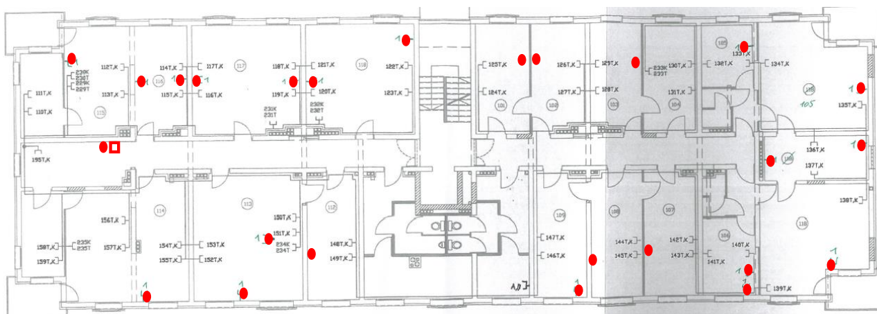
Rys.5 Schemat pomieszczeń na I piętrze z zaznaczonymi (czerwone kropki) lokalizacjami projektowanych gniazd elektrycznych i logicznych (PEL) oraz miejscem na projektowaną szafę (czerwony kwadrat).
