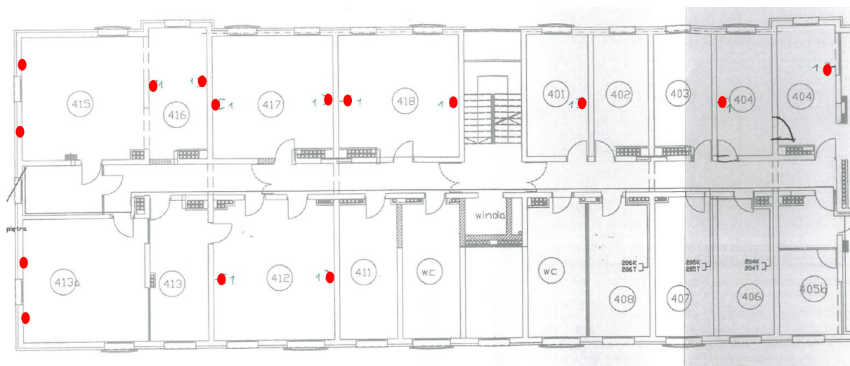
Rys.2 Schemat pomieszczeń na IV piętrze z zaznaczonymi (czerwone kropki) lokalizacjami projektowanych gniazd elektrycznych i logicznych (PEL).
