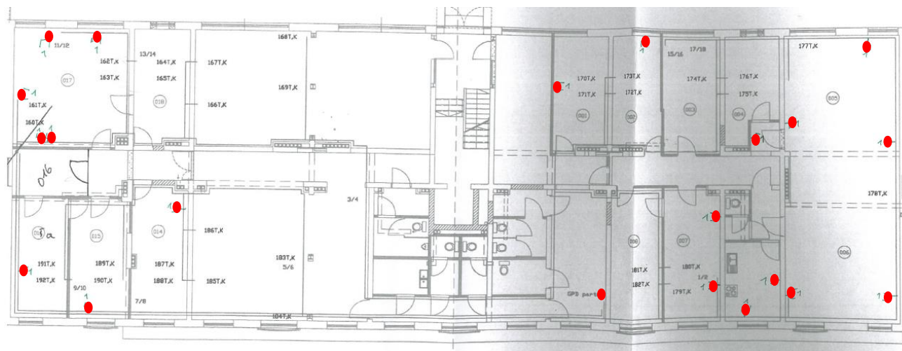
Rys.6 Schemat pomieszczeń na parterze z zaznaczonymi (czerwone kropki) lokalizacjami projektowanych gniazd elektrycznych i logicznych (PEL).
