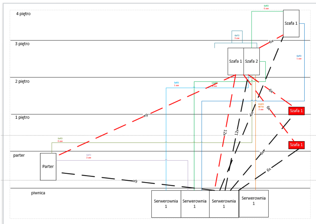
Rys.1. Schemat rozmieszczenia traktów światłowodowych istniejących (linia ciągła) wraz z proponowanymi (linia przerywana).
